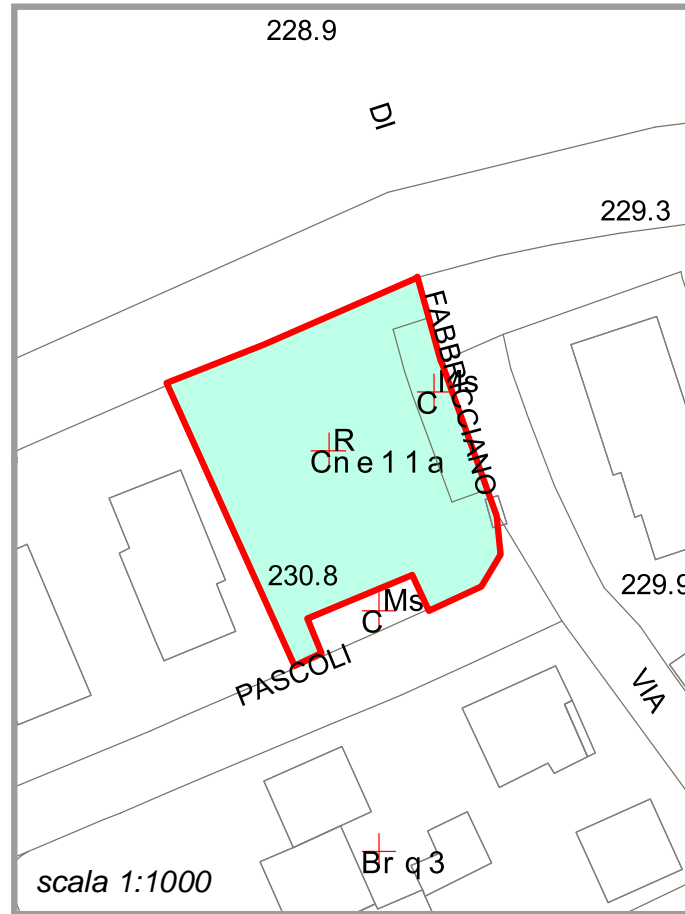
Carta della Fattibilità Idraulica Tav. 6d
