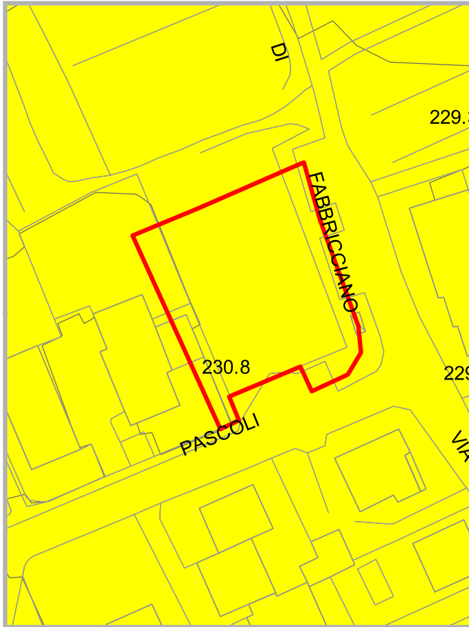
Carta della Pericolosità Geomorfologica Tav. 6a
